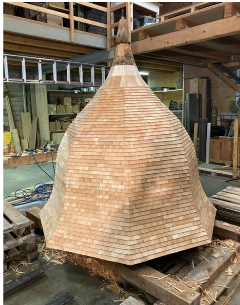
Holzschindeldeckung am Glockenturm
