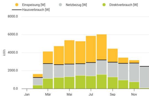
PV Jahresübersicht 2024
