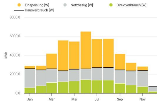
PV Jahresübersicht 2025
