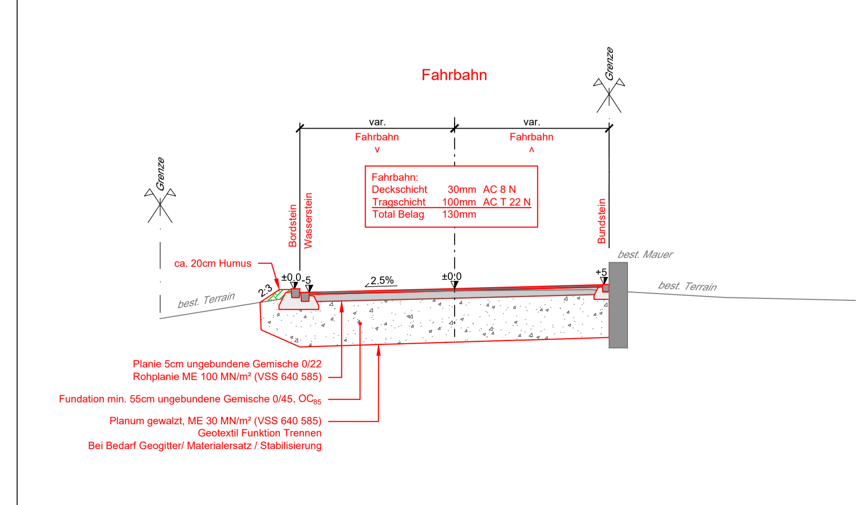
Normalprofil 1:50
